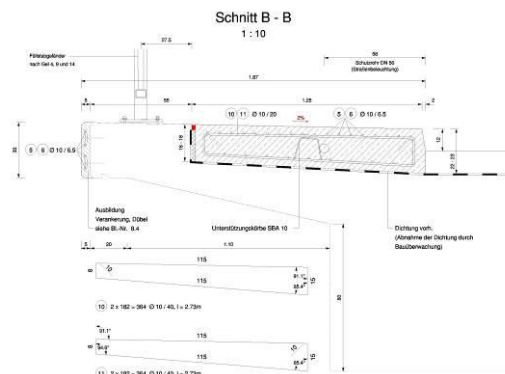
Bild 2 Schal- und Bewehrungsplan (Auszug)
