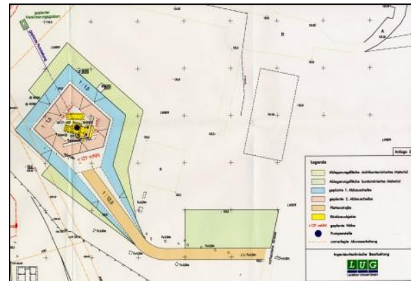
Genehmigungsplanung „Baugrube“
