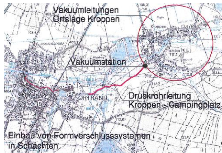
Bild 1: Planausschnitt Bearbeitungsgebiet
