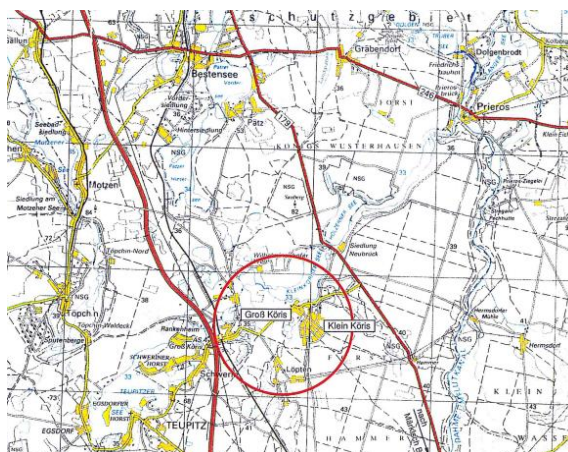
Bild 1 Planausschnitt Bearbeitungsgebiet
